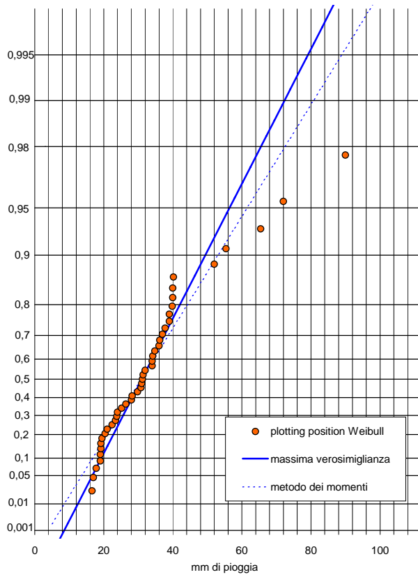
Massimi annuali delle altezze di precipitazione di durata 1 ora
